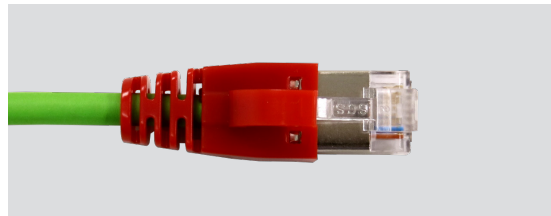
11 Connector RJ-45 (IEC 61869-10, IEC 61869-11)
